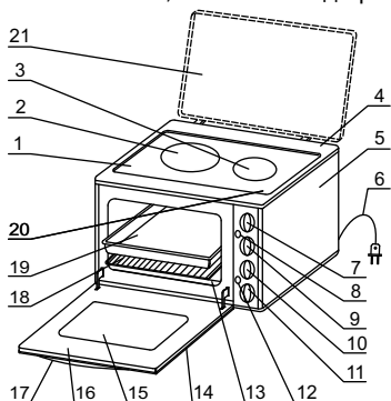
Фиг. 1 Печки модели 201VF, 201VFB, 203VF, 203VFB и модификациите им
